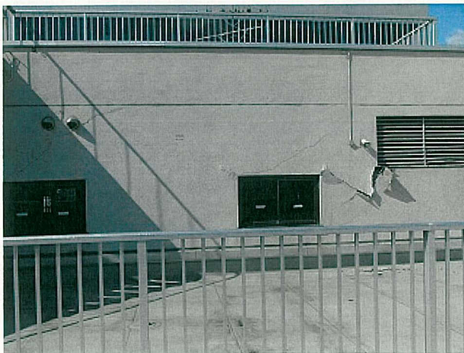
(6)会館外壁…ひび割れ多数，陥没
