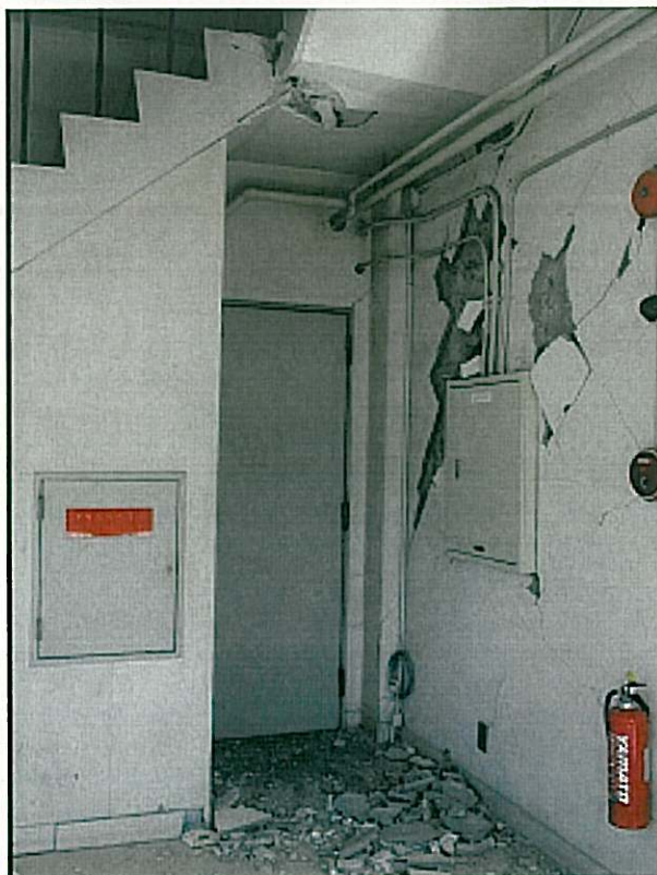
(5)屋上機械室入口…壁面崩落
